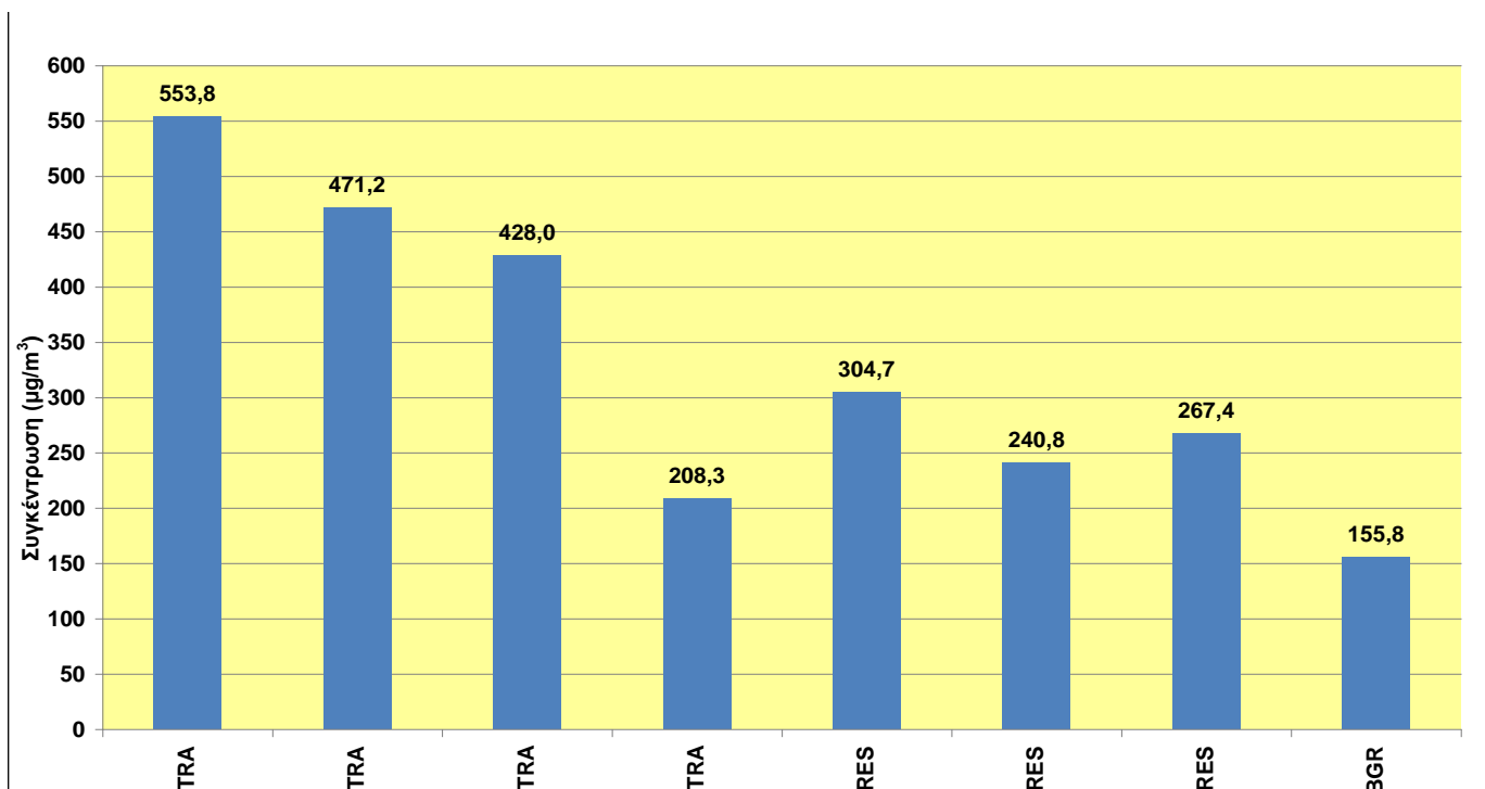
Σχήμα 10: Ετήσιοι μέσοι όροι CO για το έτος 2014 στους διάφορους Σταθμούς του Δικτύου Παρακολούθησης Ποιότητας Αέρα
