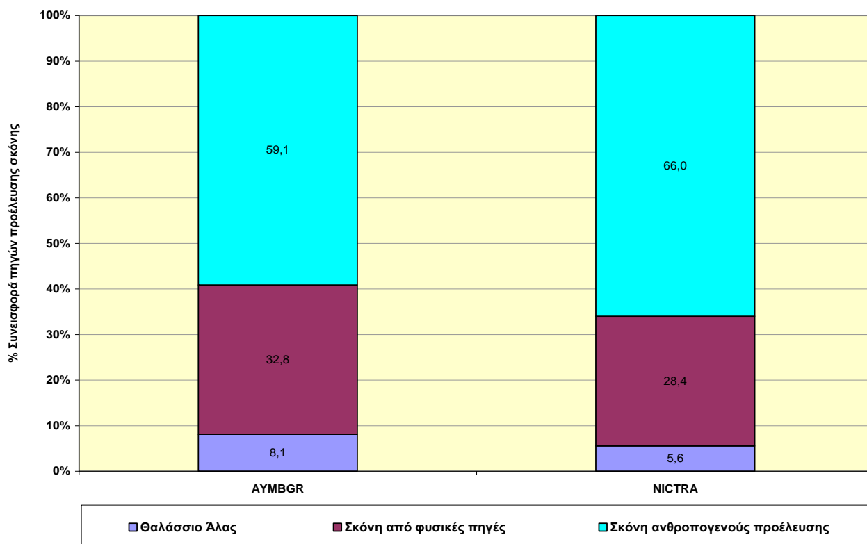
Σχήμα 19: Ποσοστό συνεισφοράς πηγών προέλευσης σκόνης για το έτος 2014 στον Σταθμό Υποβάθρου Αγίας Μαρίνας και στον Κυκλοφοριακό Σταθμό Λευκωσίας.
