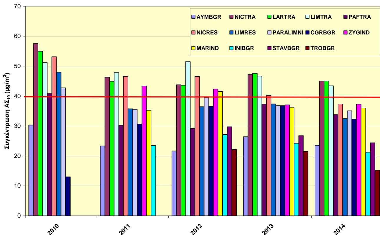
Σχήμα 13(α): Ετήσιοι μέσοι όροι ΑΣ 10 για την περίοδο 2010-2014 στους διάφορους Σταθμούς του Δικτύου Παρακολούθησης Ποιότητας Αέρα
