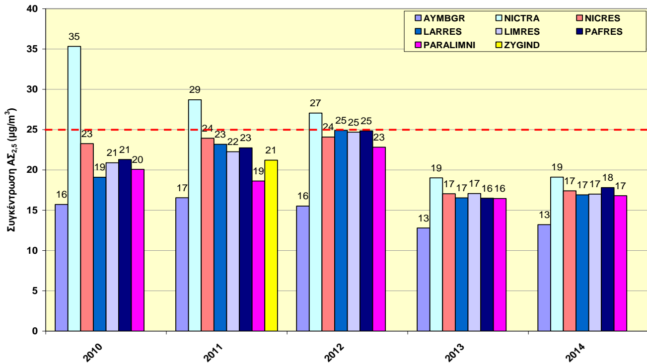
Σχήμα 14: Ετήσιοι μέσοι όροι ΑΣ_{2,5} για την περίοδο 2010-2014 στους διάφορους Σταθμούς του Δικτύου Παρακολούθησης Ποιότητας Αέρα
