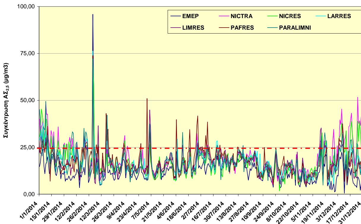
Σχήμα 16: Ημερήσια διακύμανση ΑΣ 2,5 για το έτος 2014 στους Σταθμούς του Δικτύου Παρακολούθησης Ποιότητας Αέρα.
