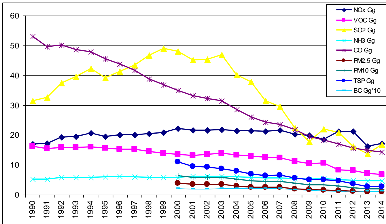
Σχήμα 20: Τάσεις εκπομπών για την περίοδο 1990-2014 (Κύριοι Ρύποι και Σωματίδια)
