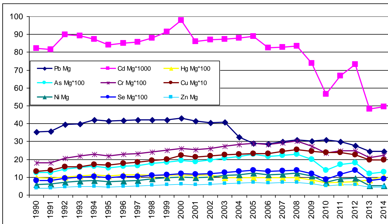
Σχήμα 21: Τάσεις εκπομπών για την περίοδο 1990-2014 (Βαρέα Μέταλλα)
