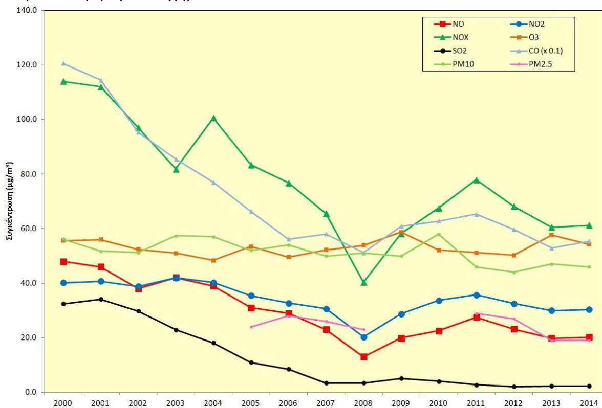
Σχήμα 3: Μέσες ετήσιες τιμές \text{NO} , \text{NO}_2 , \text{NO}_x , \text{O}_3 , \text{SO}_2 , \text{CO} , \text{A}\Sigma_{10} ( \text{PM}_{10} ) και \text{A}\Sigma_{2,5} ( \text{PM}_{2,5} ) στον Κυκλοφοριακό Σταθμό Λευκωσίας
