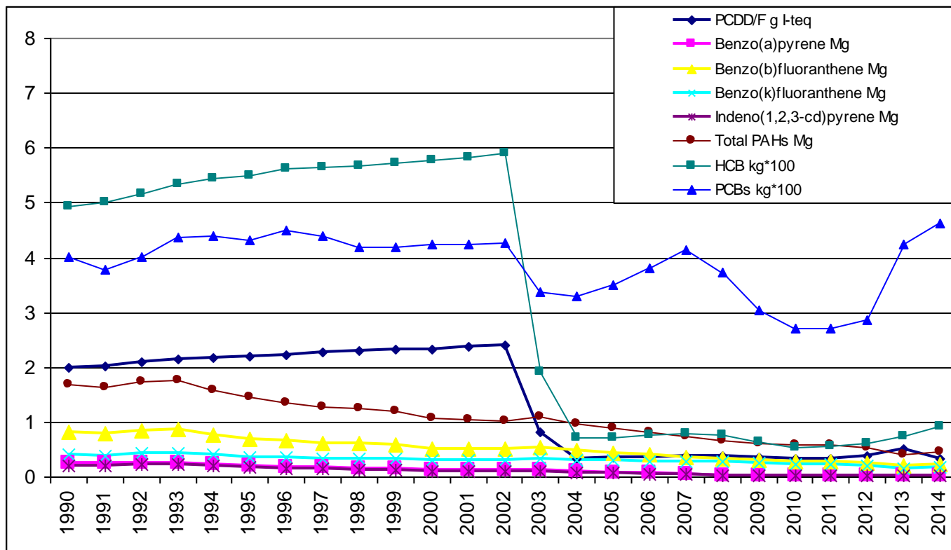
Σχήμα 22: Τάσεις εκπομπών για την περίοδο 1990-2014 (Εμμονοι Οργανικοί Ρύποι) Figure 22: Emission trends for the period 1990-2014 (Persistent Organic Pollutants)
