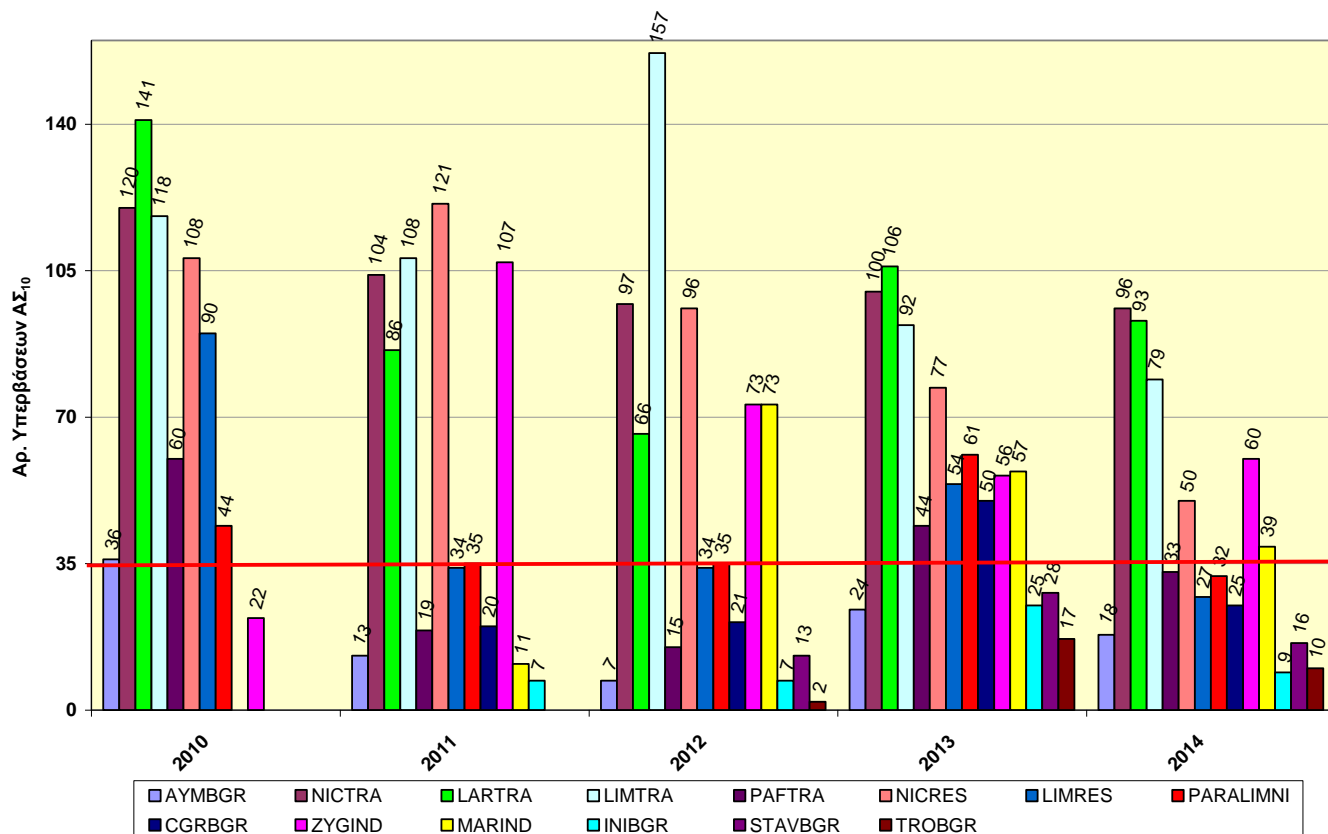
Σχήμα 13(β): Αριθμός υπερβάσεων κατ’ έτος της ετήσιας οριακής τιμής για τα ΑΣ 10 στους διάφορους Σταθμούς του Δικτύου Παρακολούθησης Ποιότητας Αέρα για την περίοδο 2010-2014.
