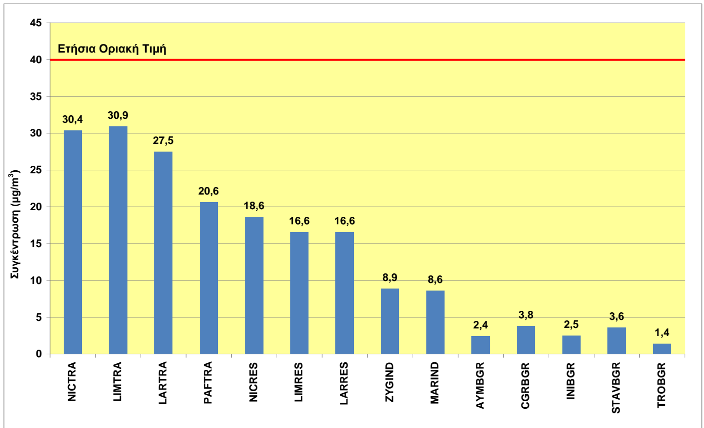
Σχήμα 4: Ετήσιοι μέσοι όροι NO 2 για το έτος 2014 Figure 4: NO 2 Annual Mean Concentration for 2014
