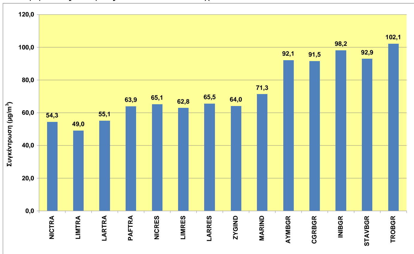
Σχήμα 7: Ετήσιοι μέσοι όροι O_3 για το έτος 2014 στους διάφορους Σταθμούς του Δικτύου Παρακολούθησης Ποιότητας Αέρα
