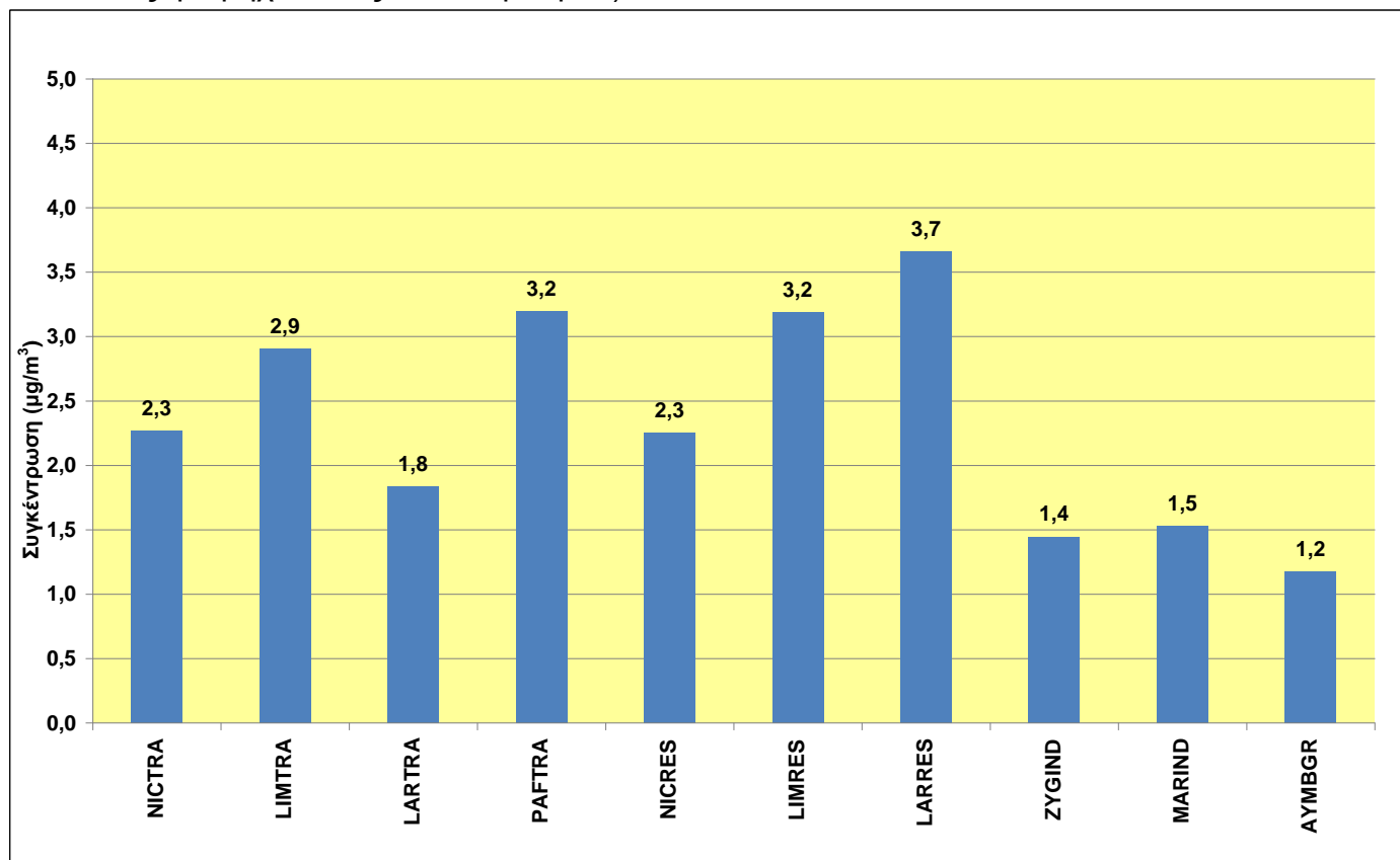
Σχήμα 6: Ετήσιοι μέσοι όροι SO 2 για το έτος 2014 στους διάφορους Σταθμούς του Δικτύου Παρακολούθησης Ποιότητας Αέρα
